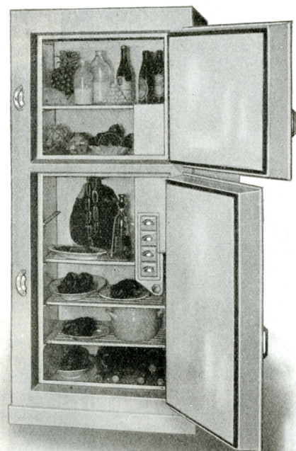
Kylskåp för hushållsbehov enligt Platens och Munters system. Ur Teknisk Tidskrift, 1925, utgiven av STF.
